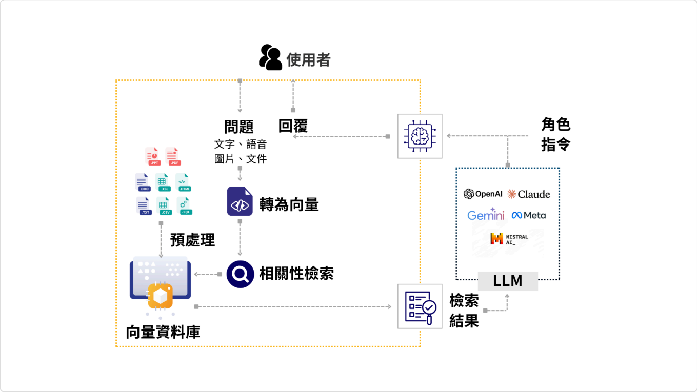
RAG 流程
